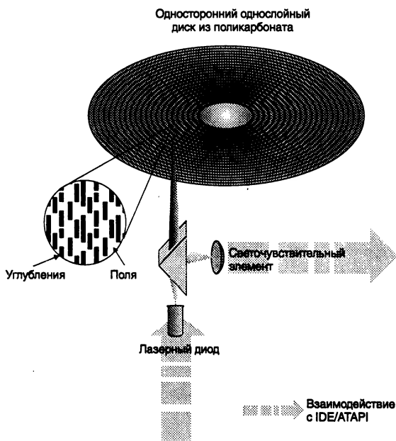
Рис. 3.3. Принцип действия дисководов CD-ROM
