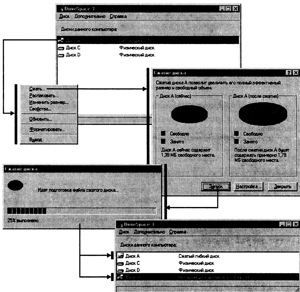
Рис. 14.10. Схема применения технологии уплотнения дисков
