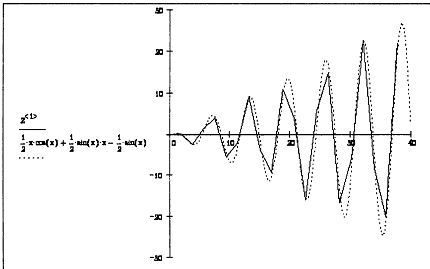
Рис. 18.7. Графики численного и точного решения дифференциального уравнения
